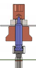
DUDOR NÉLKÜLI, ROSSZ MINŐSÉGŰ CSAVARANYA
