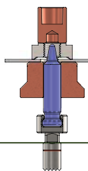
ROSSZUL TÁJOLT LEMEZ
