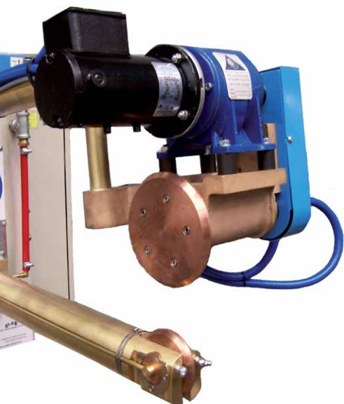
HOSSZIRÁNYÚ HEGESZTÉS
